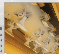
Rotore Ø 325 mm con martelli Rotor Ø 325 mm avec marteaux Rotor Ø 325 mm with hammer blades Rotor Ø 325 mm mit Hammerschaufeln Rotor Ø 325 mm con martillos
