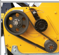
Tendicinghia automatico e sistema di ingrassaggio centralizzato Tendeur de courroie automatique et graissage centralisé Automatic belt tightener and centralized greasing Automatischer Riemenspanner und Zentralschmierung Tensor automático de correa y sistema de engrase centralizado
