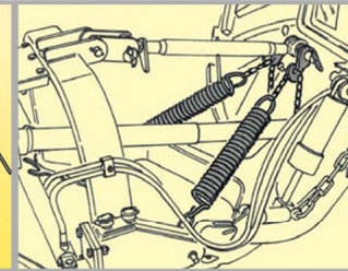
Kit molle per frontale Kit ressort pour frontal Spring kit for front Federsatz für Frontanbau Kit resortes para enganche delantero
