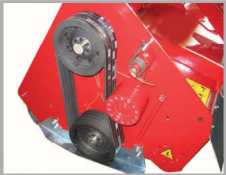
Tendinghia automatico Tendeur de courroie automatique Automatic belt tightener Automatischer Riemenspanner Tensor de correa automático
