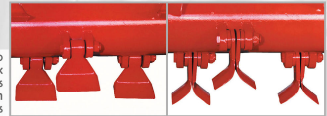
Coltelli a Y Fléaux Y Y-flails Y-Messer Cuchillas Y
