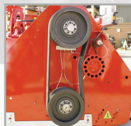
Tendinghia automatico Tendeur de courroie automatique Automatic belt tightener Automatischer Riemenspanner Tensor de correa automático
