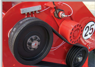
Tendicinghia automatico Tendeur de courroie automatique Automatic belt tightener Automatischer Riemenspanner Tensor de correa automático
